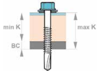
schroef zonder ring
